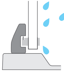
Профіль в нижній частині душової кабінки: 10°, Nexty, Pivot, Blix Slim, Blix, Supernova
