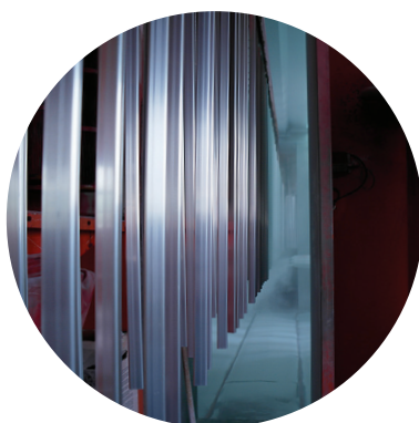
Фарбувальний цех RAVAK Електростатичне нанесення порошкової фарби на алюмінієві профілі душових кабін, дверей і штор для ванн.
